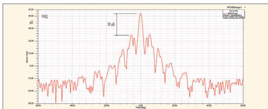
Рис. 8. Сечение ДН, решение методом физической оптики
